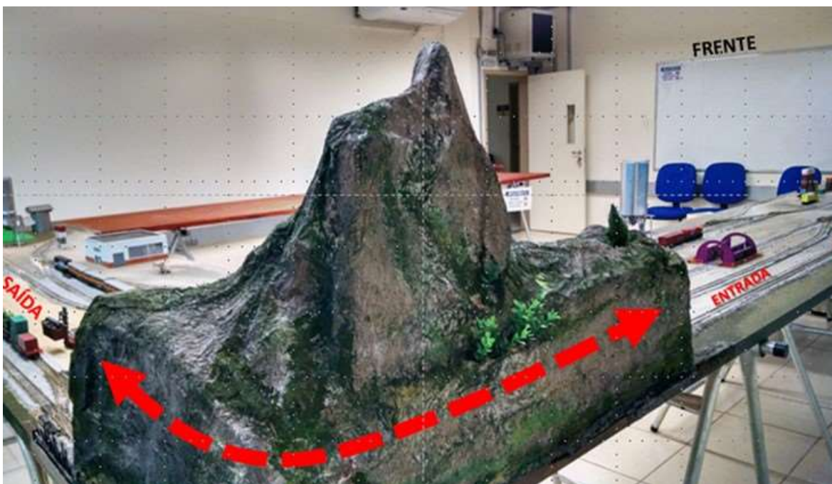
Figura 7.35 — Detalhe atrás da montanha: arranjo de canto para aproveitar espaço.
